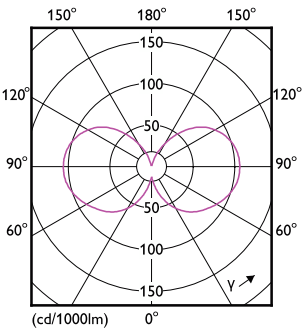
LEDbulb MAS EU A60 4W E27 830 CL-LDD
